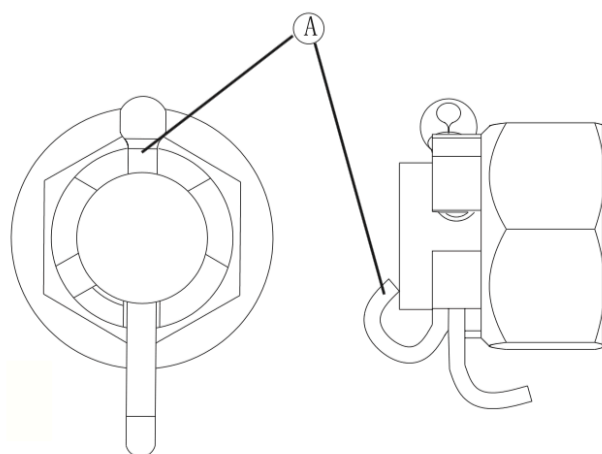
Ⓐ Závlačka
